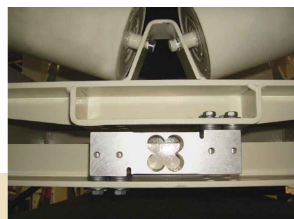
sistema de pesaje individual con celdas de carga centralizada
